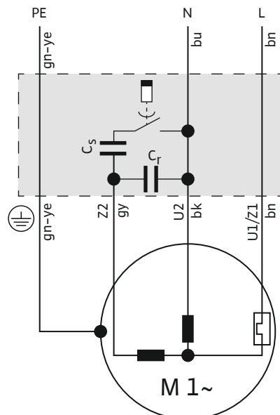
Fig. 4: Схемa на свързване 1~ мотор
