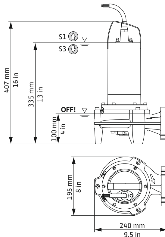
Fig. 3: Монтажни размери
