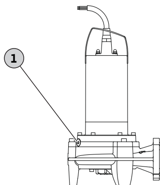
Fig. 6: Смяна на маслото в уплътнителната камера
