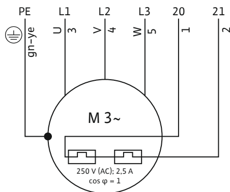
Fig. 5: Схемa на свързване 3~ мотор
